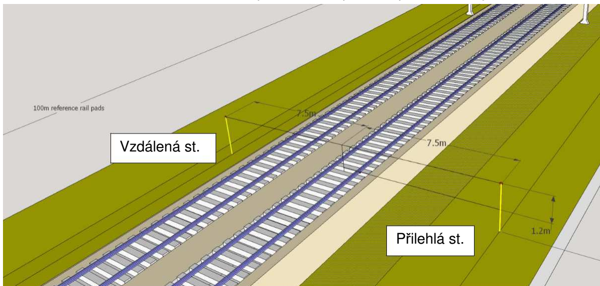
Obrázek 3: Umístění mikrofónu
