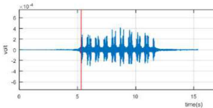
Zrychlení měřené na kolejnici (akcelerace): Úsek S2
