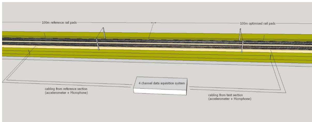
Obrázek 6: Instalace vybavení a kabeláže
