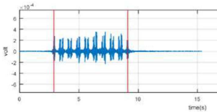
Zrychlení měřené na kolejnici (akcelerace): Úsek S1
