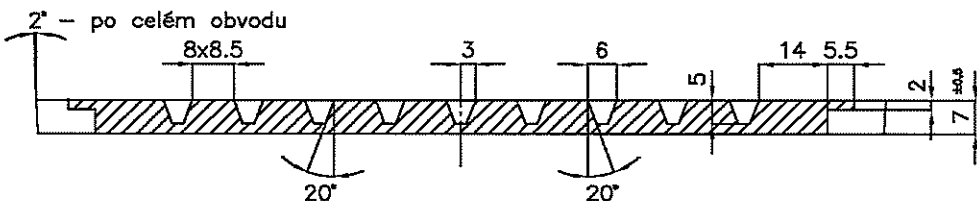
Obr.2 Příčný řez A - A
