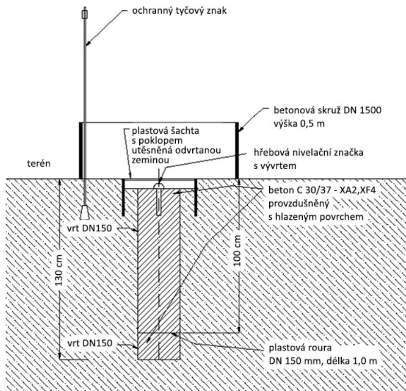
Schéma základní odlehčené stabilizace bodu
