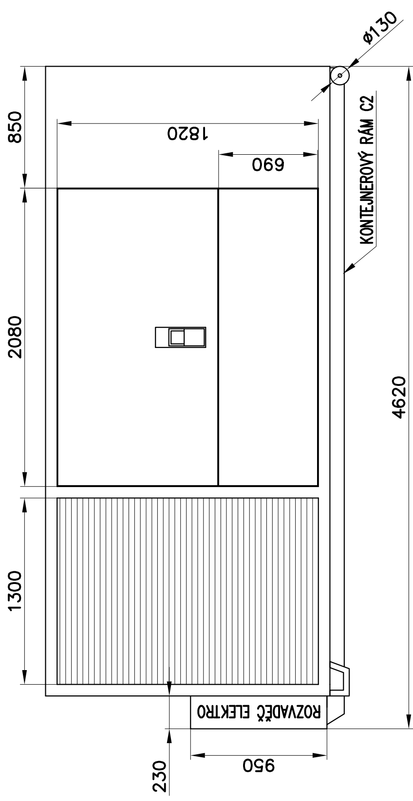
BOČNÍ POHLED – LEVÁ STRANA
