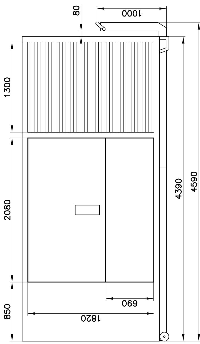
BOČNÍ POHLED – PRAVÁ STRANA
