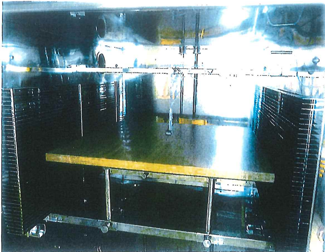
Foto 1 -- Zkušební vzorek - DTD laminovaná, dezén ořech Lyon, dekór č.: 9614 PS, uložený v klimatizační komoře VOC TEST 1000
