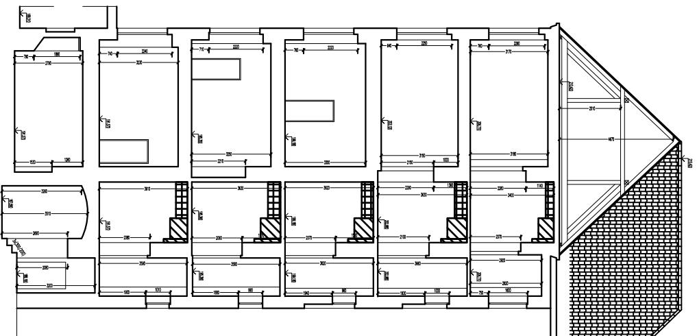
ŘEZ 3-3 SCHEMA
