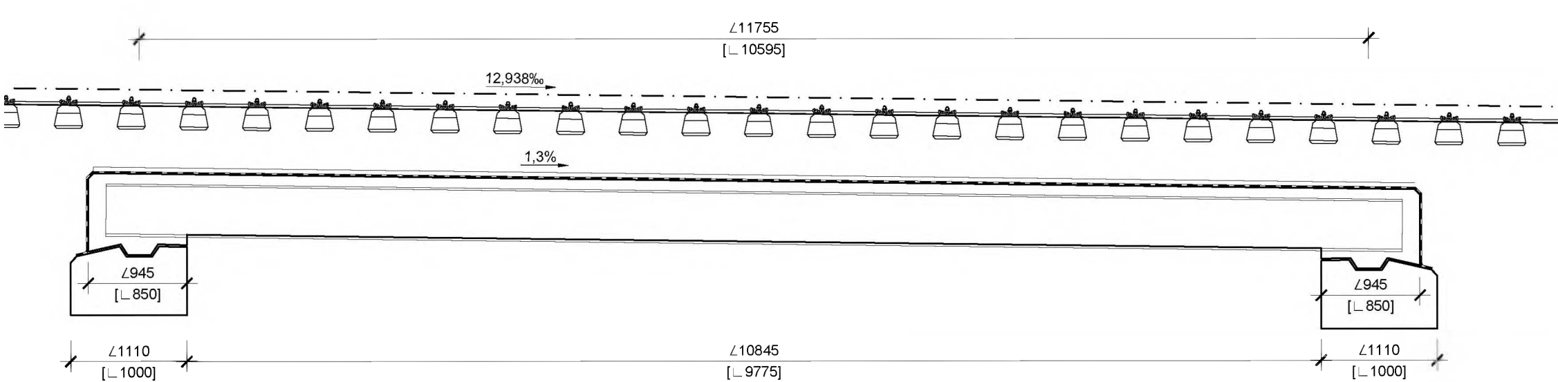
PODÉLNÝ ŘEZ M 1:50
