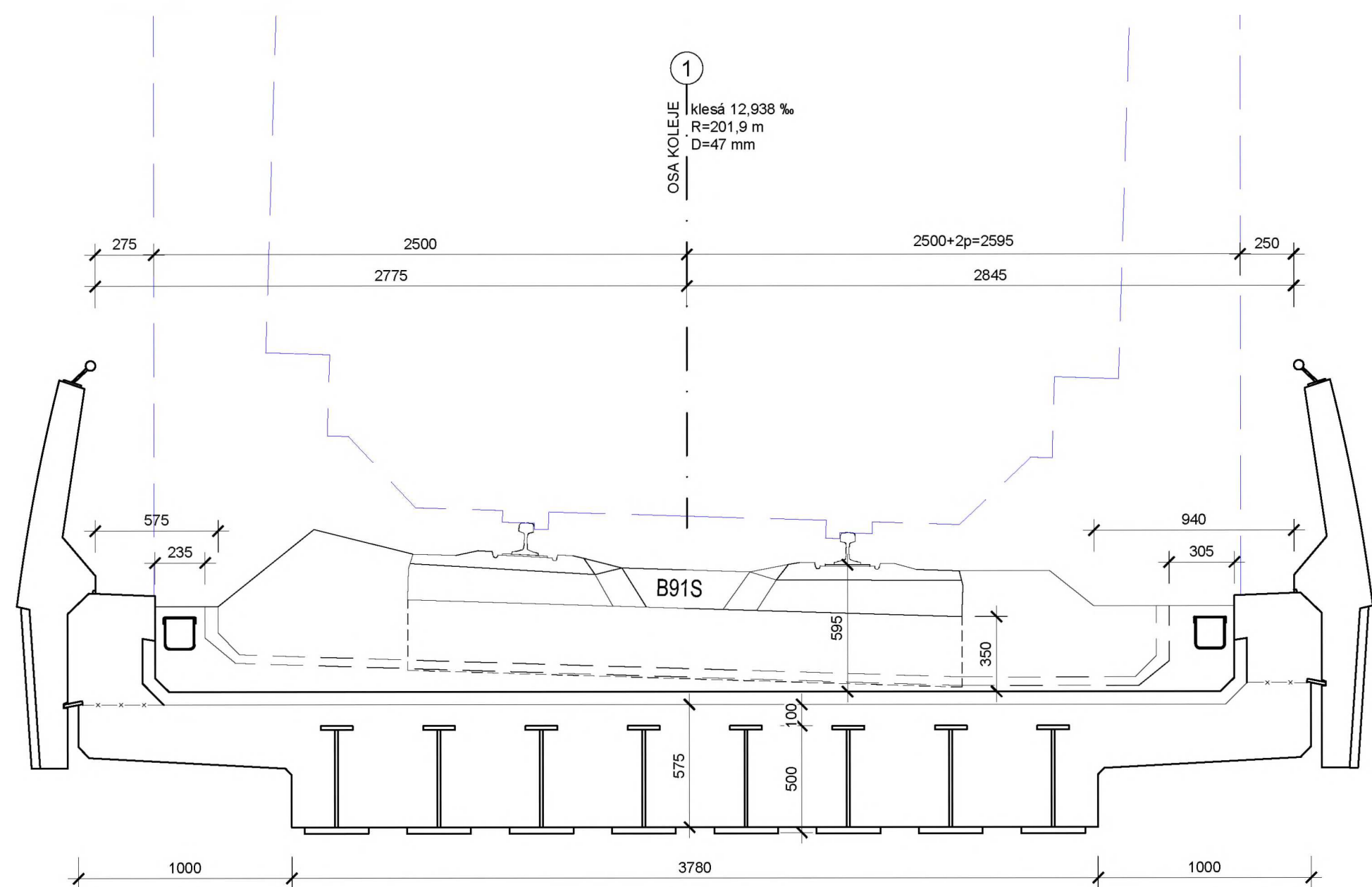
VZOROVÝ PŘÍČNÝ ŘEZ M 1:25
