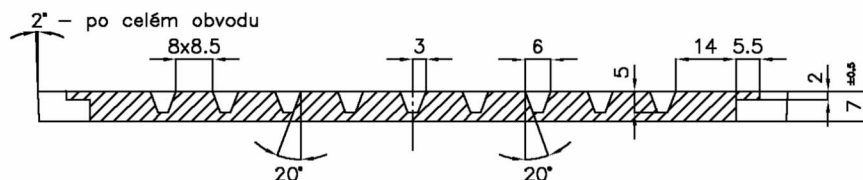
Obr.2 Příčný řez A - A
